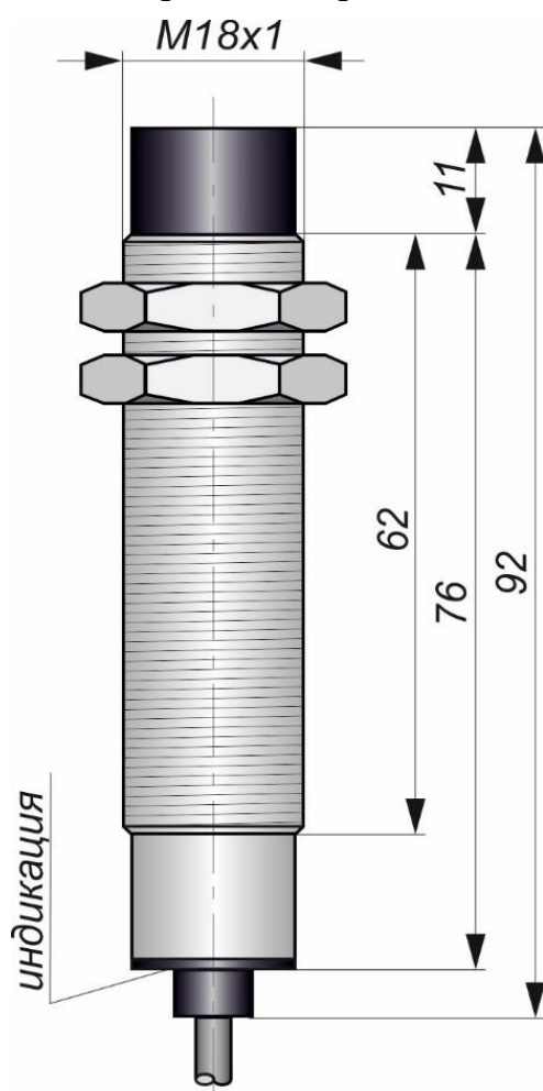
Габаритный чертеж
